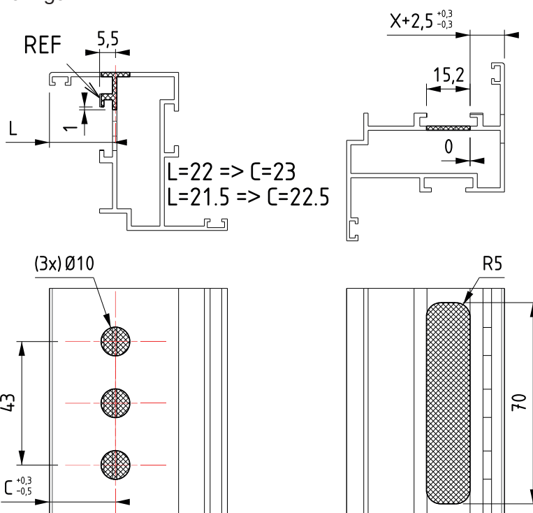
Uitfrezingen
