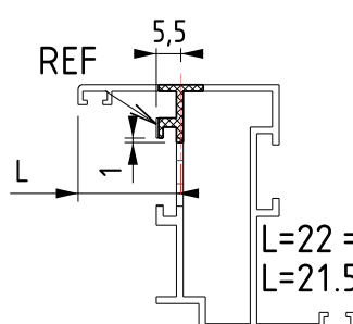
Uitfrezingen
