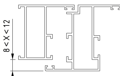
Profielafmeting
