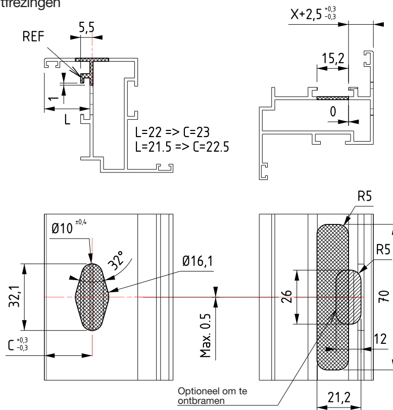
Uitfrezingen
